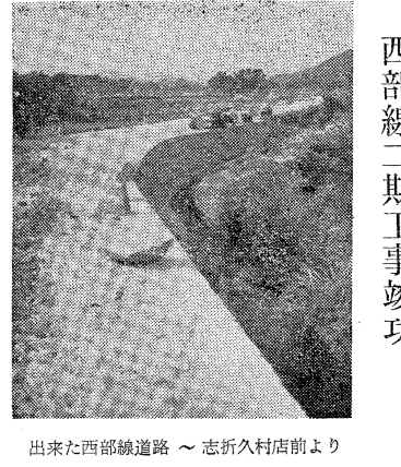
出来た西部線道路 ~ 志折久村店前より
