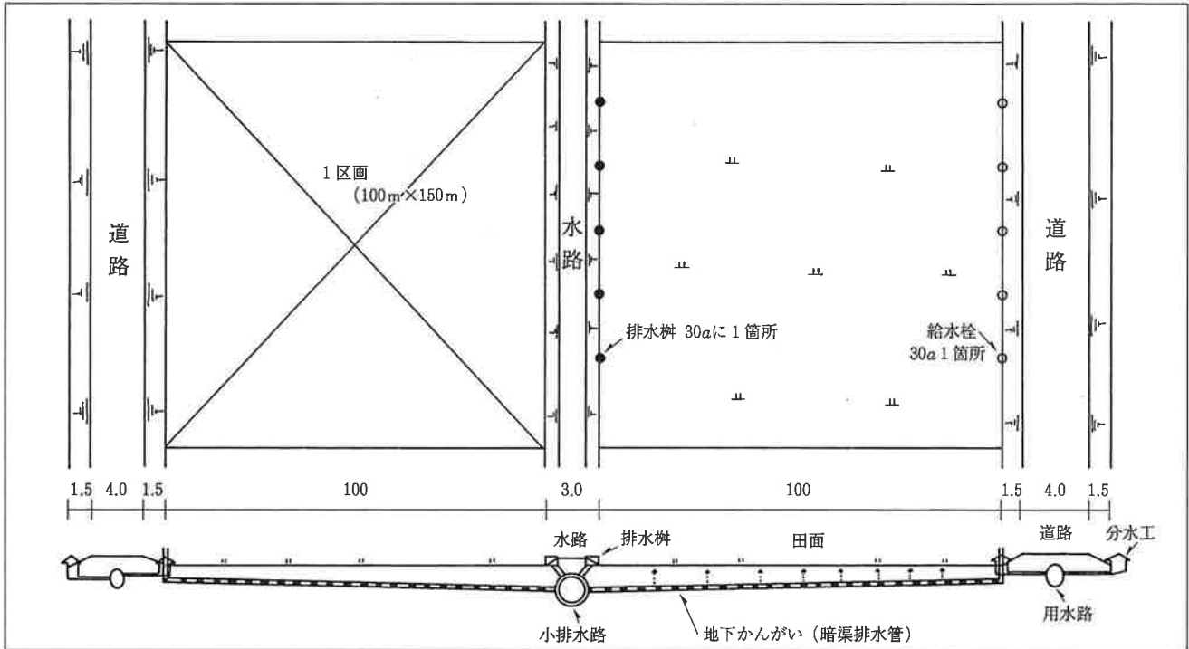
▼一区画平面・断面図
