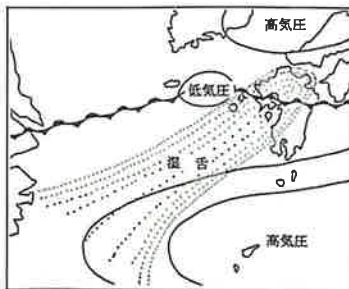
集中豪雨型の気圧配置
