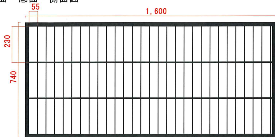
天面・底面・側面図
