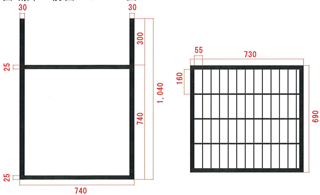
前面(扉)・前面フレーム図
