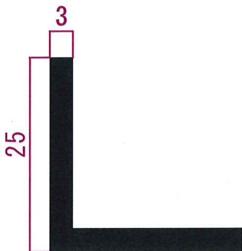
Lアングル (3*25mm等辺)
