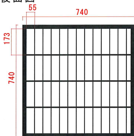
後面図
